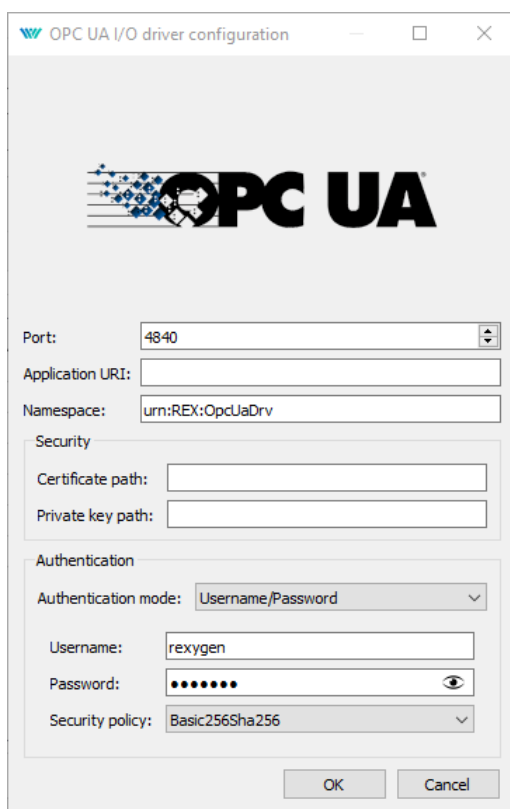
Obrázek 2.4: Konfigurace ovladače v módu OPC UA Server
